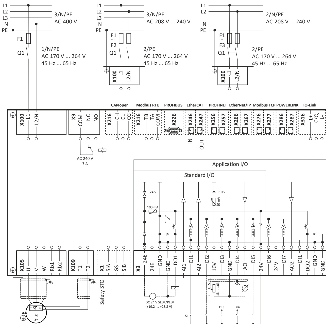
Fig. 3: Wiring example
